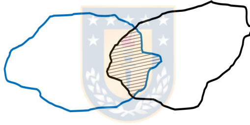
Figura 2.4: Esquema que representa \Omega_1 (en azul), \Omega_2 (en negro) y la región donde interactúan \tilde{\Omega} (achurada)
