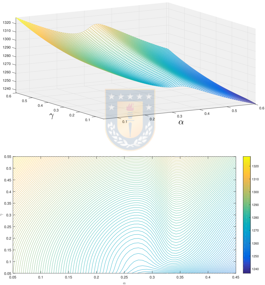
Figura 7.34: Gráfico sup.: Tridimensional, Gráfico inf.: Líneas de Contorno.
