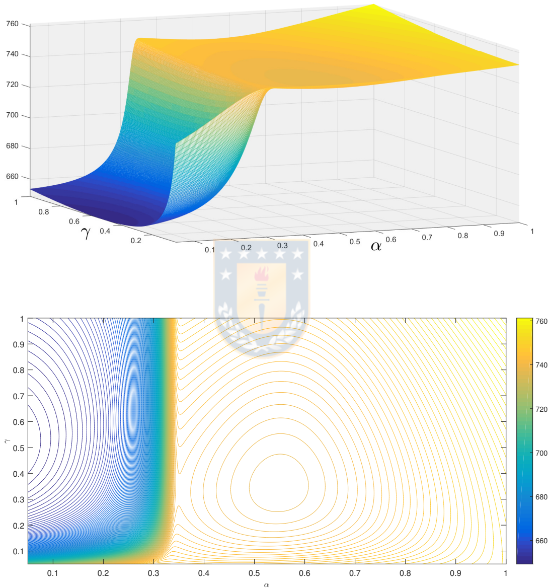
Figura 7.14: Gráfico sup.: Tridimensional, Gráfico inf.: Líneas de Contorno.
