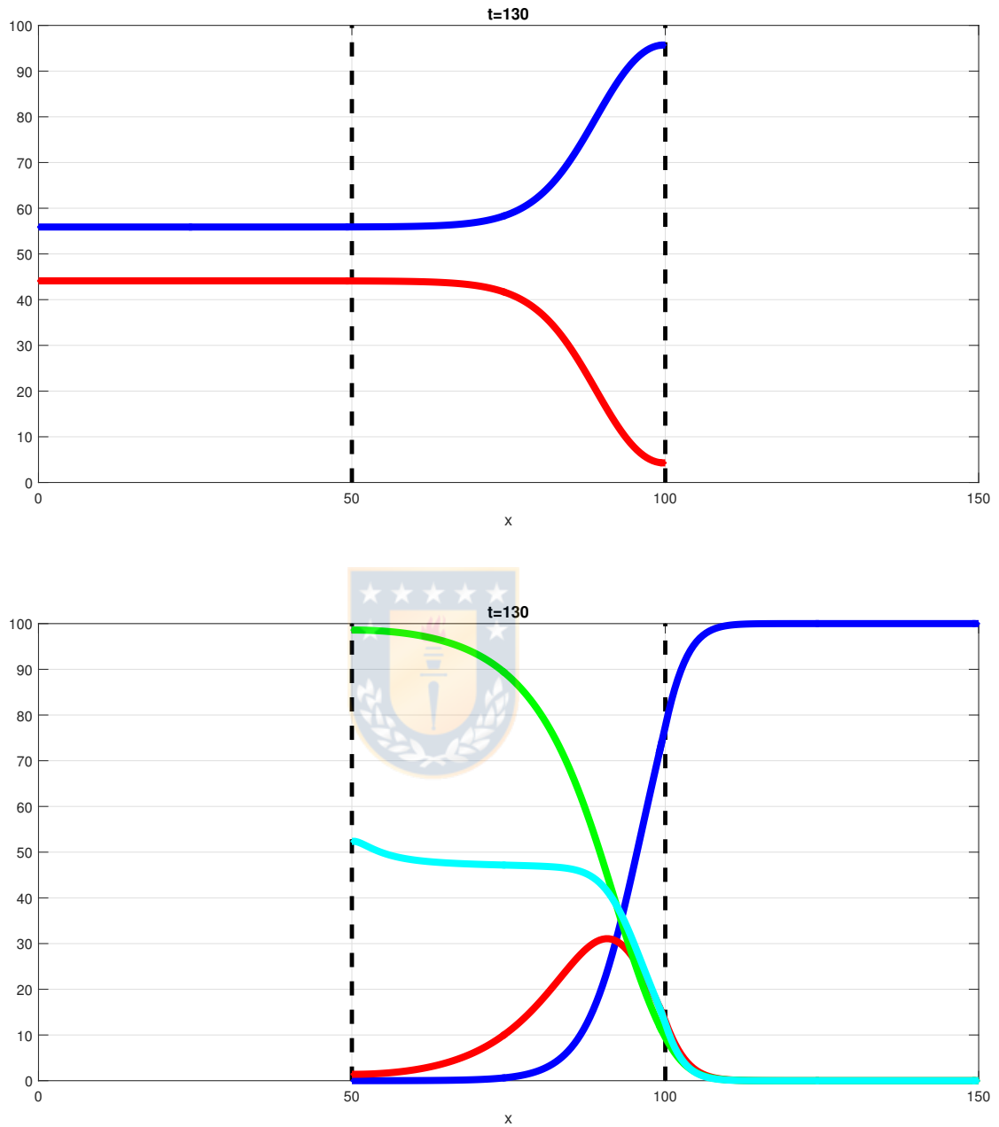
Figura 7.21: Solución en t = 130 . Gráfico sup.: u_1 en azul y u_2 en rojo; Gráfico inf.: v_1 en azul, v_2 en rojo, v_3 en verde y c en celeste.
