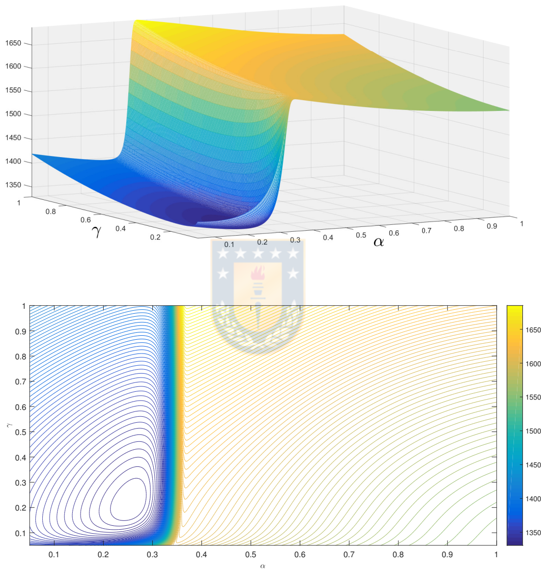
Figura 7.15: Gráfico sup.: Tridimensional, Gráfico inf.: Líneas de Contorno.
