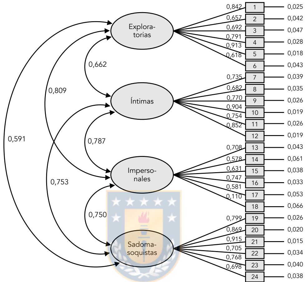
Figura 1. Análisis factorial confirmatorio para la escala WSFQ considerando un modelo de cuatro factores (modelo A).
