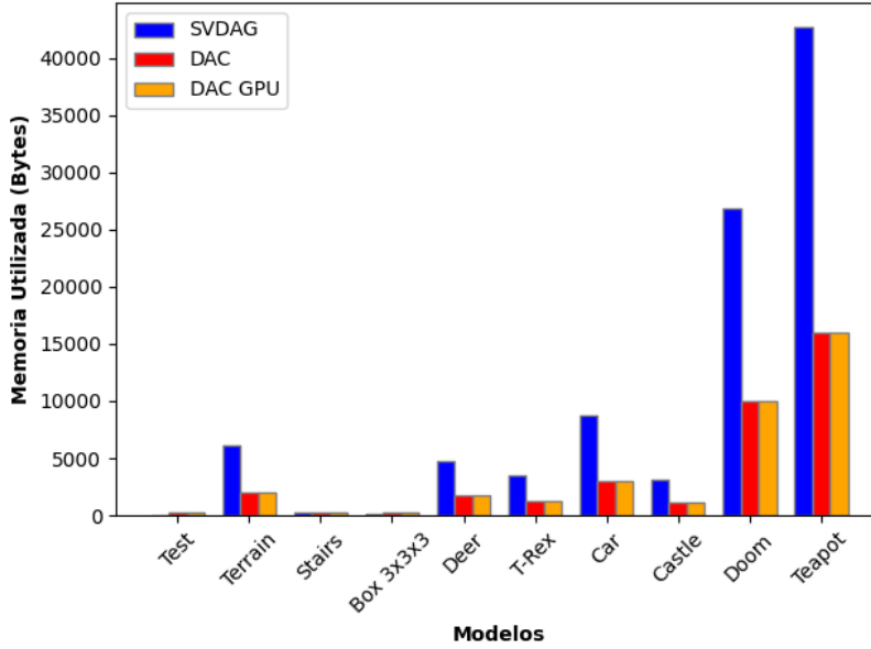
Figura 12: Comparación del uso en memoria de cada estructura de datos por modelo
