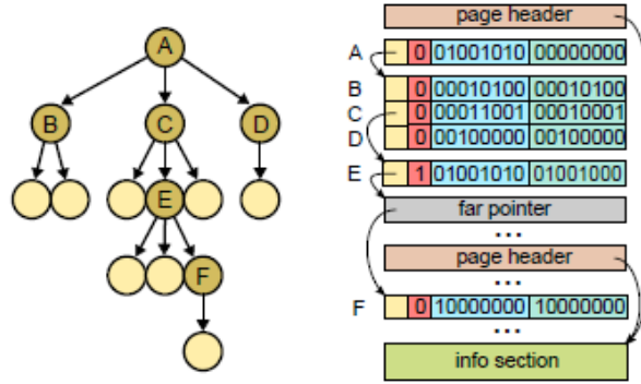
Figura 8: Izquierda: ejemplo de jerarquía de los voxeles. Derecha: ejemplo de arrays representando a los hijos, hay un array por cada voxel no hoja
