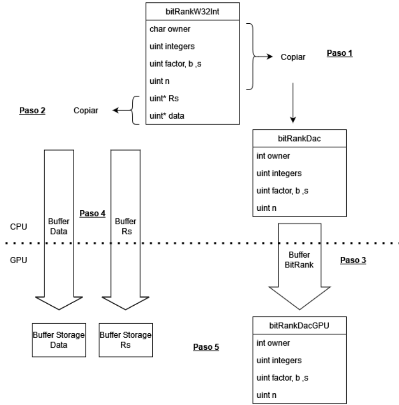
Figura 10: Diagrama explicando el paso de datos. Paso 1 : copia de datos para la nueva estructura; Paso 2 : copia de Rs y data a buffers; Paso 3 : paso de datos del buffer de bitrank a GPU; Paso 4 : paso de datos de los buffers data y Rs a GPU; y Paso 5 : Buffer Storage de data y Rs, más la estructura creada en GPU bitRankDacGPU , reciben los datos para ser utilizados en GPU
