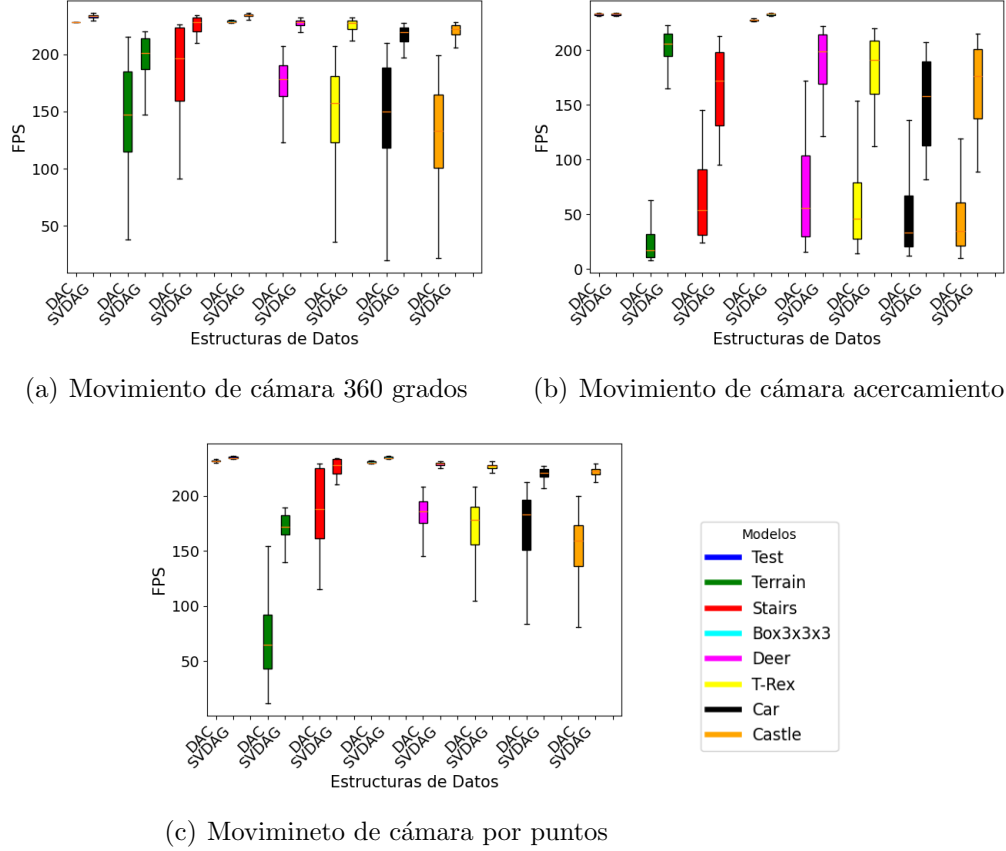
Figura 11: Experimentos de los 3 movimientos de camara automatizados sobre el dataset
