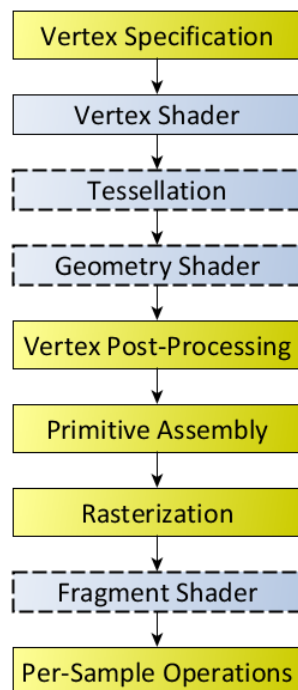
Figura 5: Ejemplo del pipeline de renderización [4]
